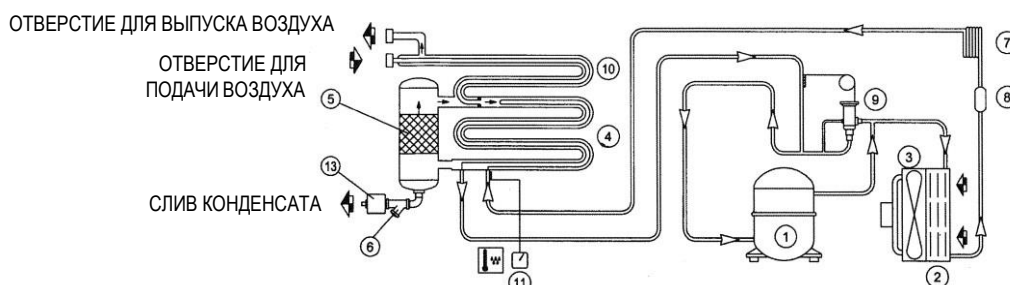
СХЕМА ОСУШИТЕЛЯ
