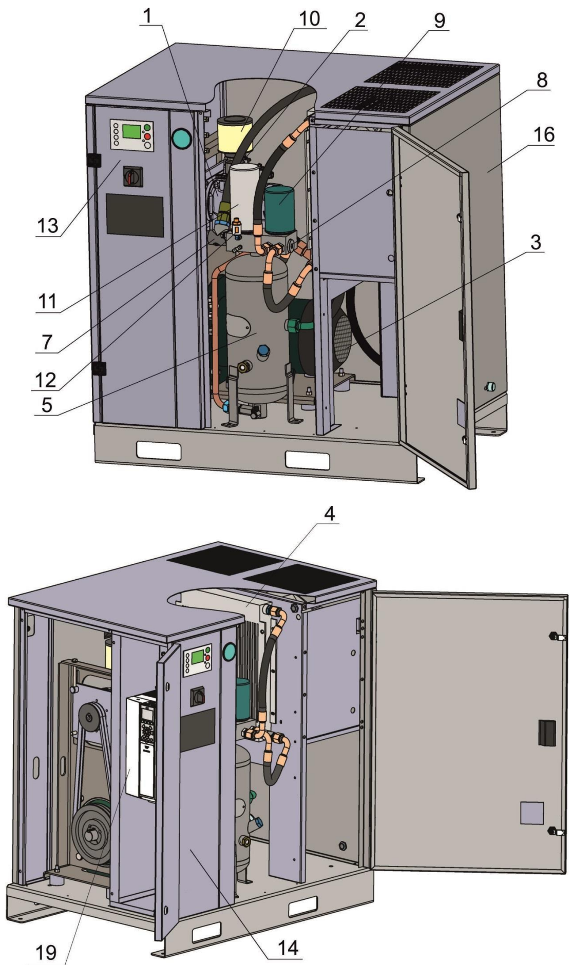
Рисунок 1 – Общий вид компрессорной установки ВК15Е-...(BC), ВК20Е-...(BC)
