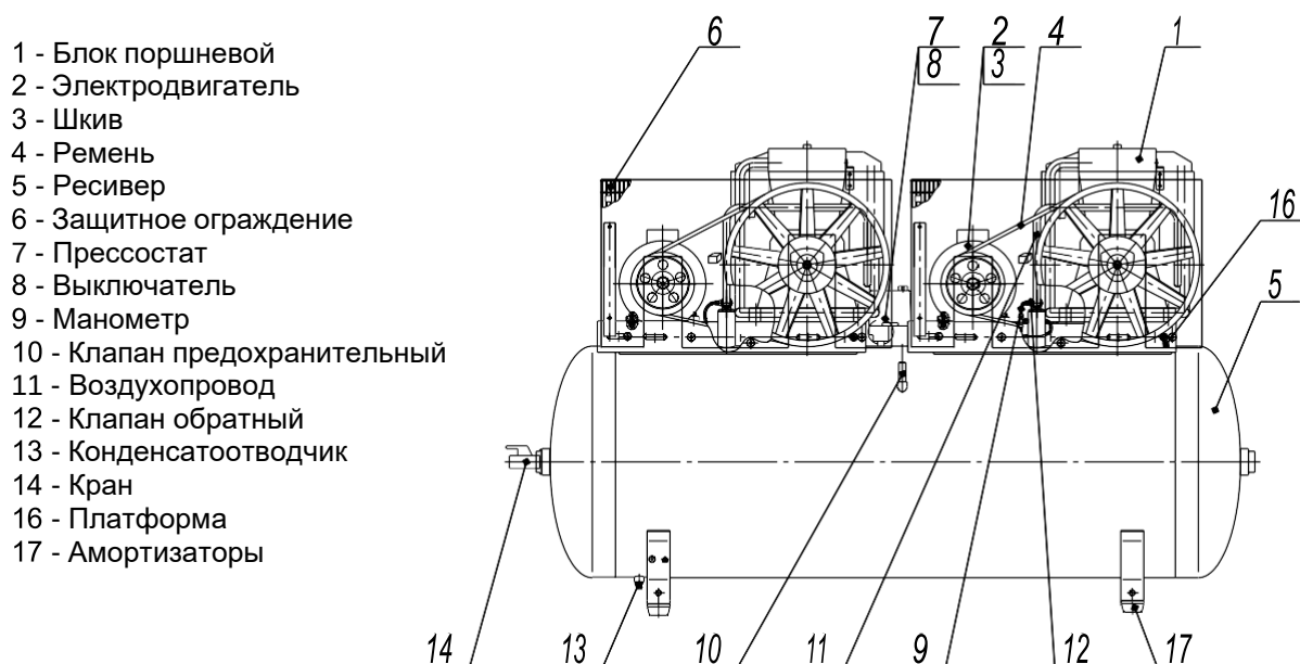
Рисунок 9 - Общий вид компрессора СБ4/Ф-500.АВ678ТБ
