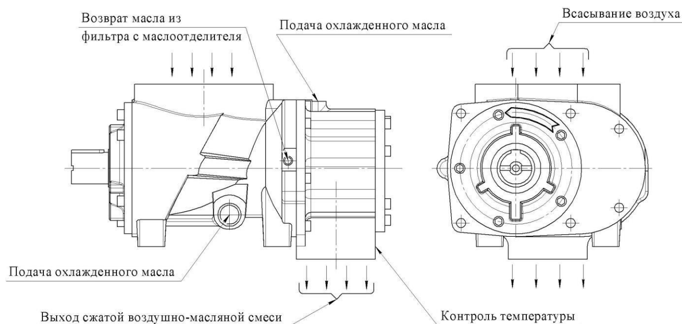
Общий вид винтового блока OS110:
